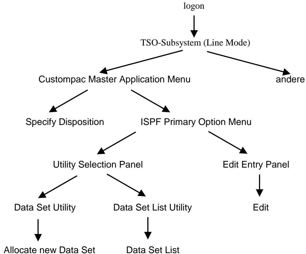
Abbildung 8: Funktionen unter TSO und ISPF
